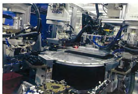
基于Super Trak的柔性装配检测线
